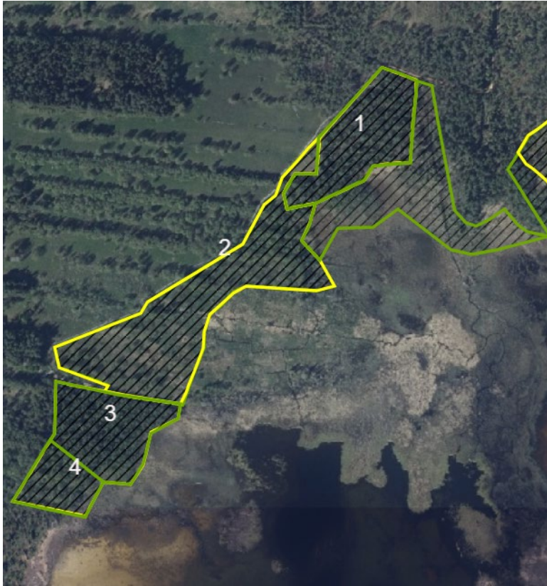
Ortofoto över det västra området av Tysjöarna med fyra fotopunkter.
